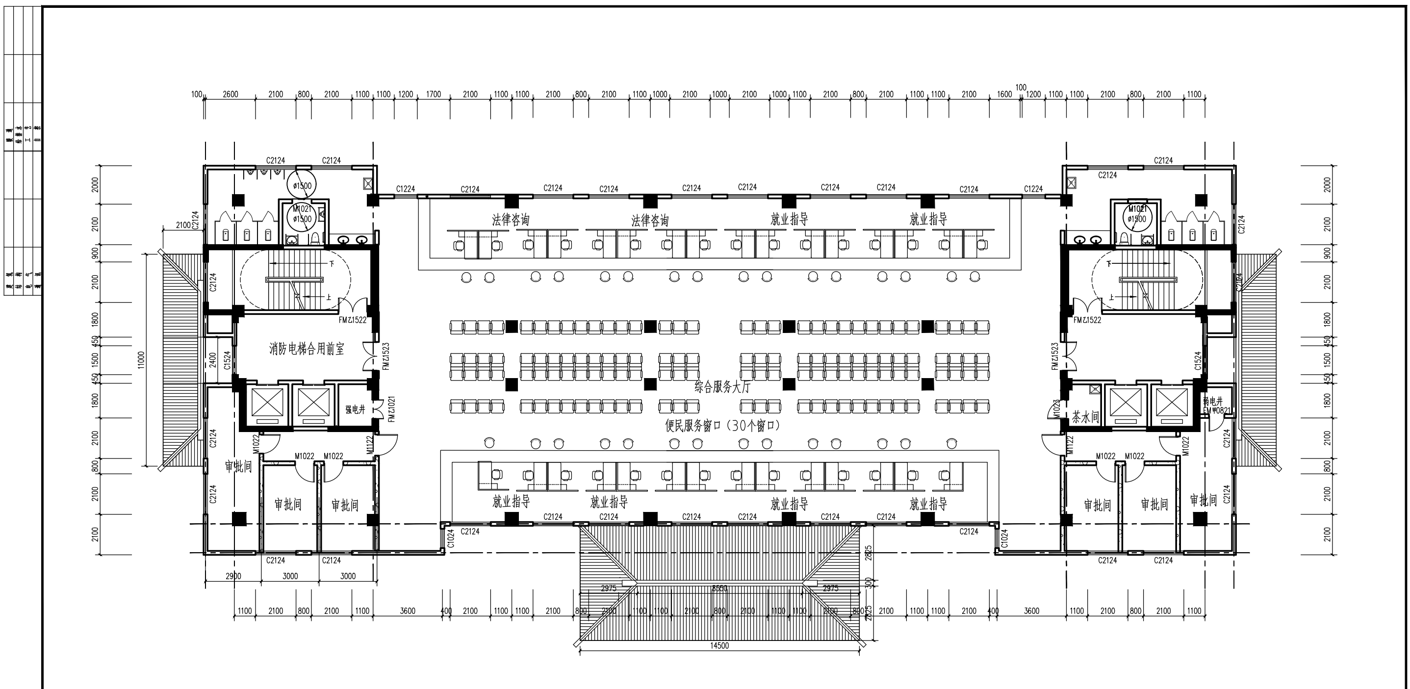
二层平面图 1:100 本层建筑面积: 978.9平米
