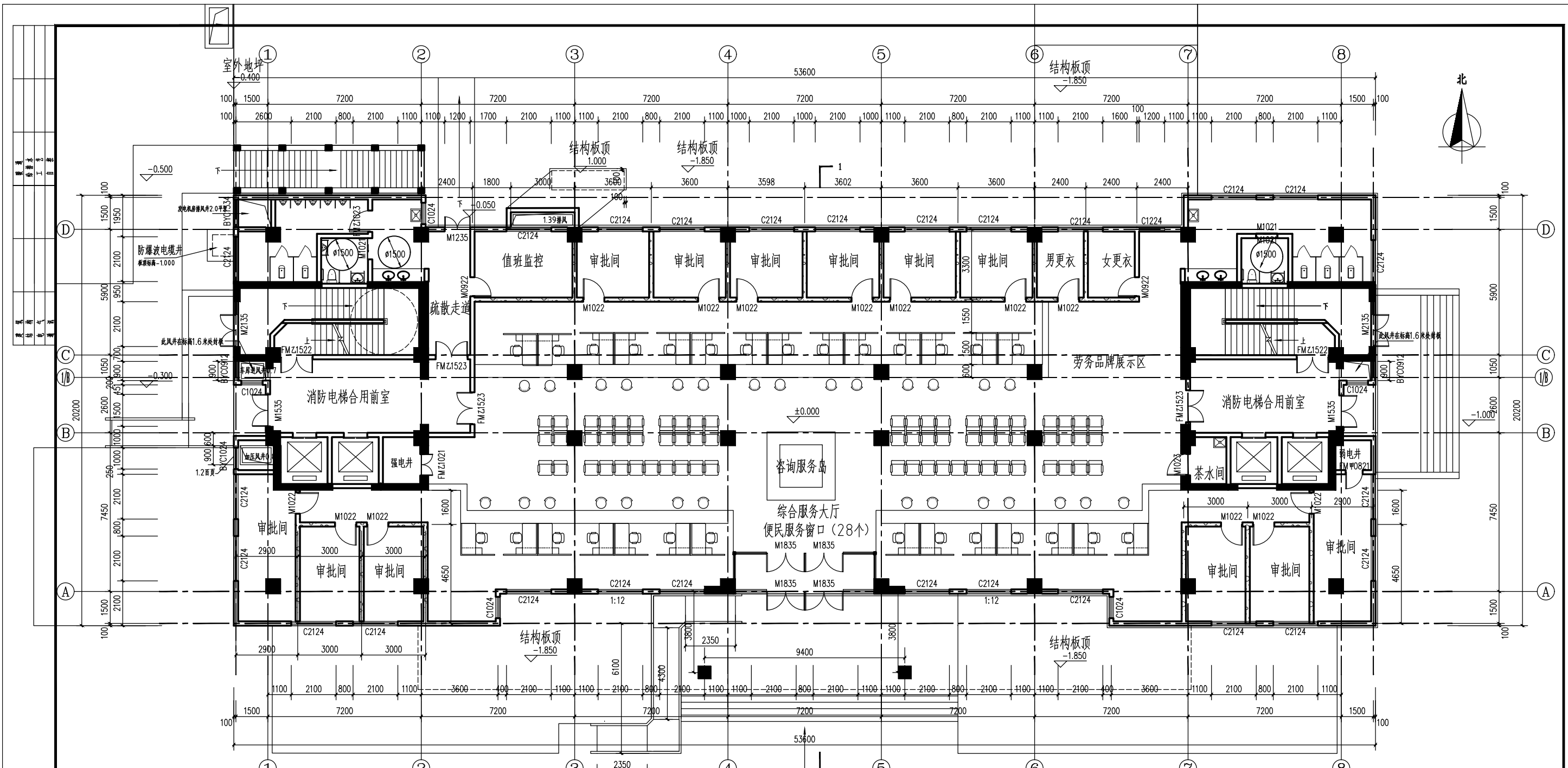
一层平面图 1:100 本层建筑面积: 978.9平方米
